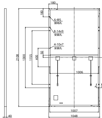
背面图
