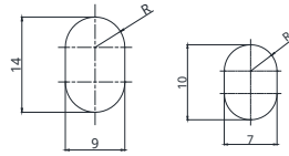
安装孔
